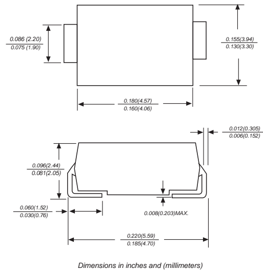
DO-214AA
